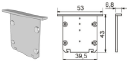
550-585-xx Embout de finition
